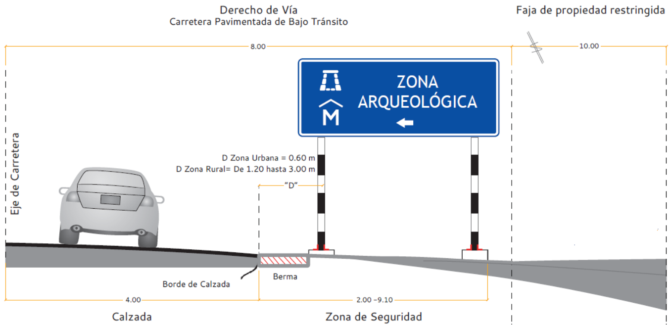
Gráfico No. 05 Gráfico del derecho de vía, zona de seguridad y faja de propiedad
