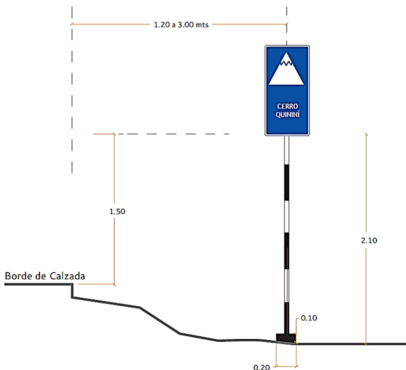
Gráfico No. 08 Señalización para zona rural
